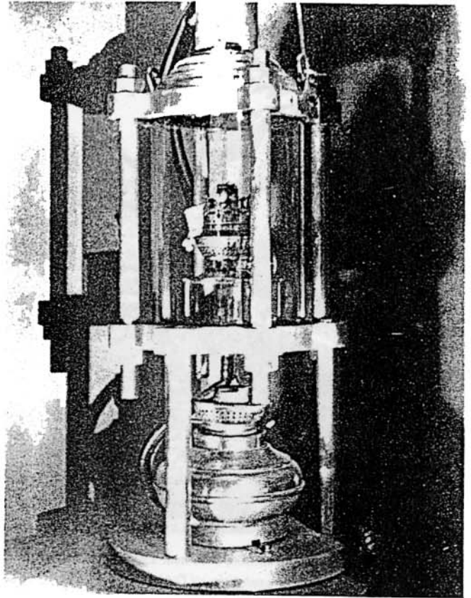
Lampe à pétrole sous-marine dont la flamme est alimentée en air par un petit détendeur branché sur le réservoir d'air sous pression (reproduction R. Stémit)
